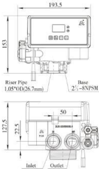
F117Q1 structure chart:
