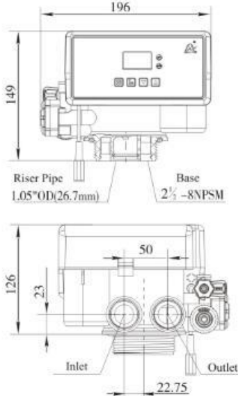
F68Q1 structure chart:
