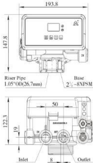
F117Q1 structure chart:
