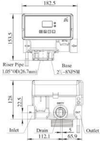
F68Q1 structure chart:
